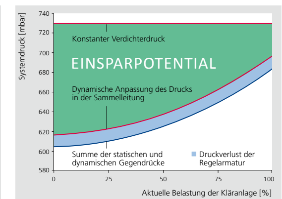
Gleitdruckregelung (mit VACOMASS® econtrol)
