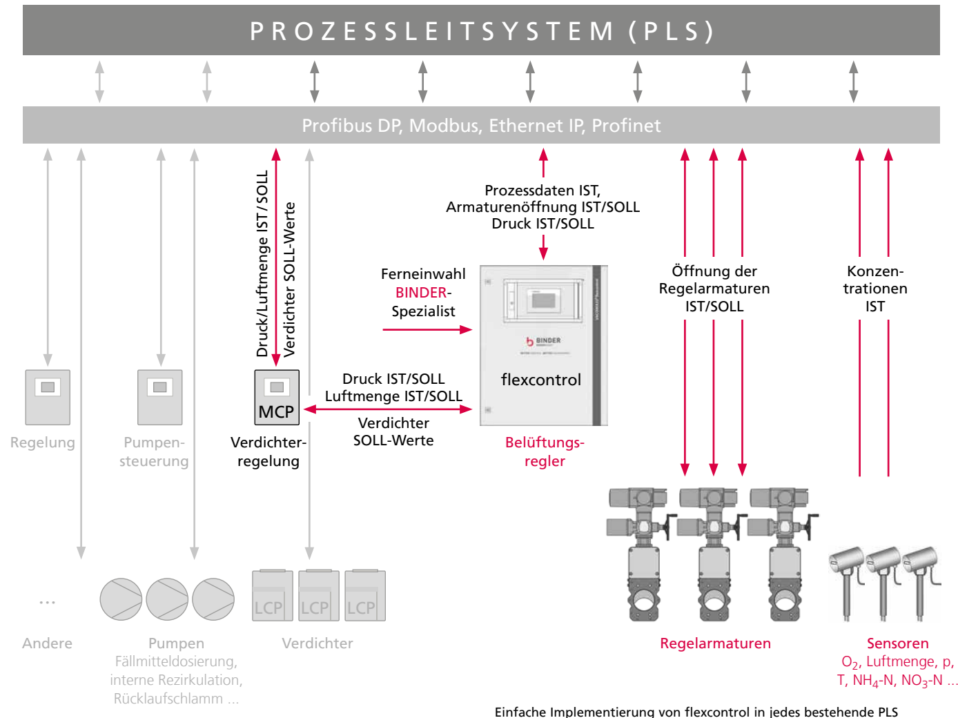
Einfache Implementierung von flexcontrol in jedes bestehende PLS
