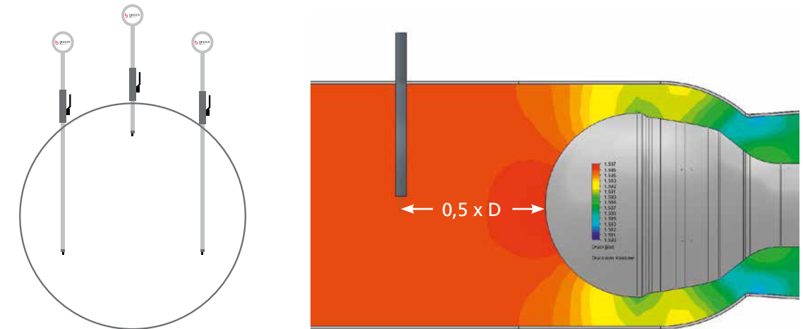
Die Grafik links oben zeigt die Anordnung mehrerer flow Sensoren in einer Sammelleitung DN800. Dadurch können auch bei relativ kurzen Einlaufstrecken in großen Nennweiten akzeptable Genauigkeiten erzielt werden.
