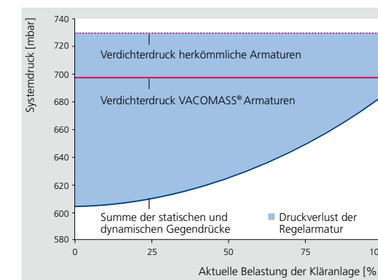
Konstantdruckregelung (ohne VACOMASS® econtrol)
