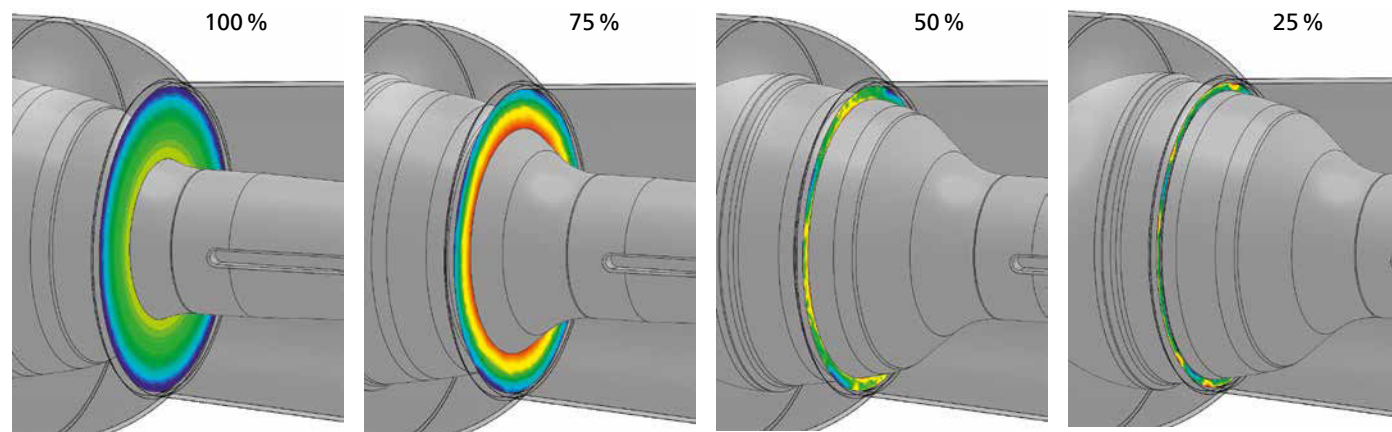
3D-Design: ein überproportionaler Anstieg der durchströmten Fläche über den Hub erzeugt eine linearisierte Betriebskennlinie
