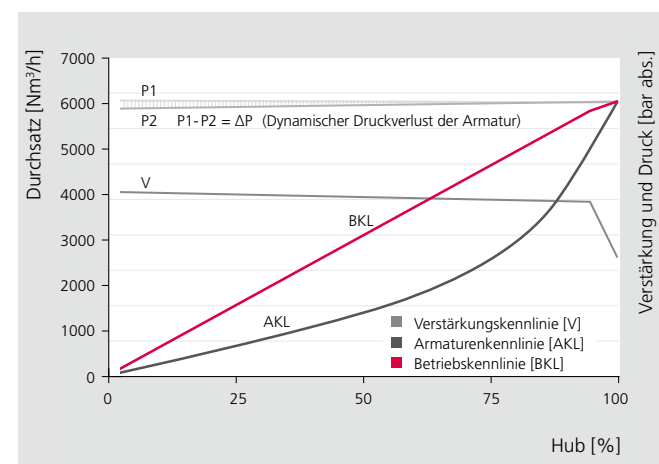
Kennlinien VACOMASS® jet control valve
